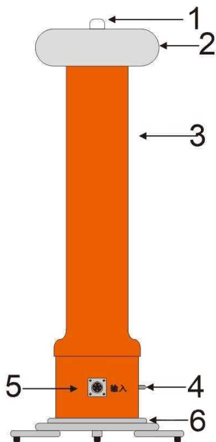
图3 倍压筒示意图
