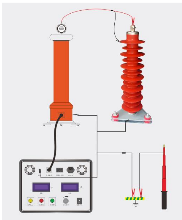
图 4 氧化锌避雷器接线图
