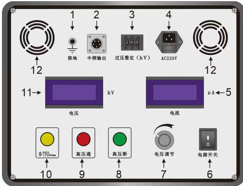
图2 面板布局图
